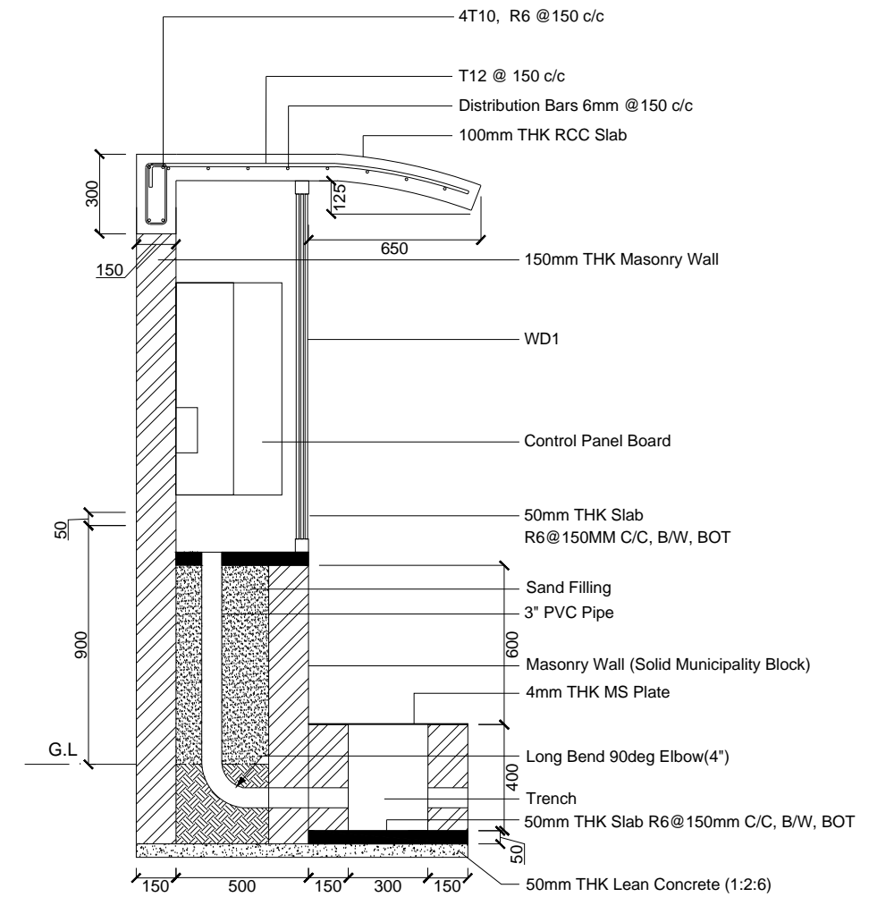
SECTION B-B SCALE: 1:25
